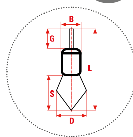
PL10 punta 30° INOX / S. Steel
